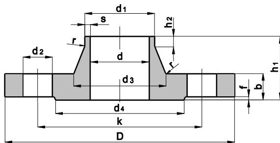
Privarovacia príruha krková PN40 DIN 2635 STN 13 11 60-11
