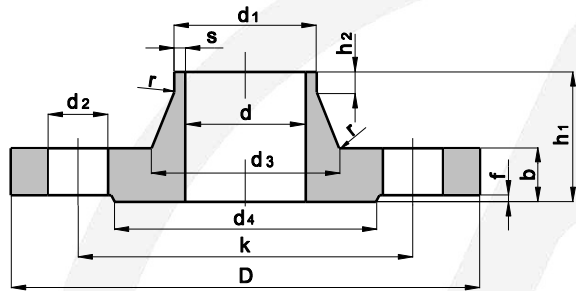
Privarovacia príruha krková PN16 DIN 2633 STN 13 11 60-11
